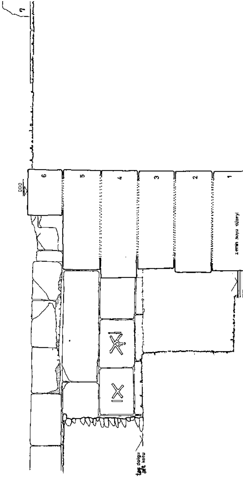
Plan : 2 — Smintheion, cella - naos içi sondajı 1985.
